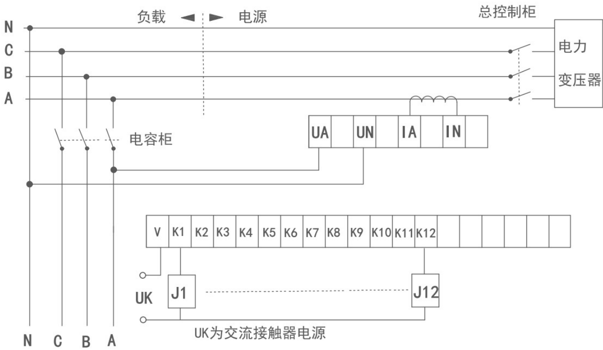
接线图 1 (取样电压 220V)
