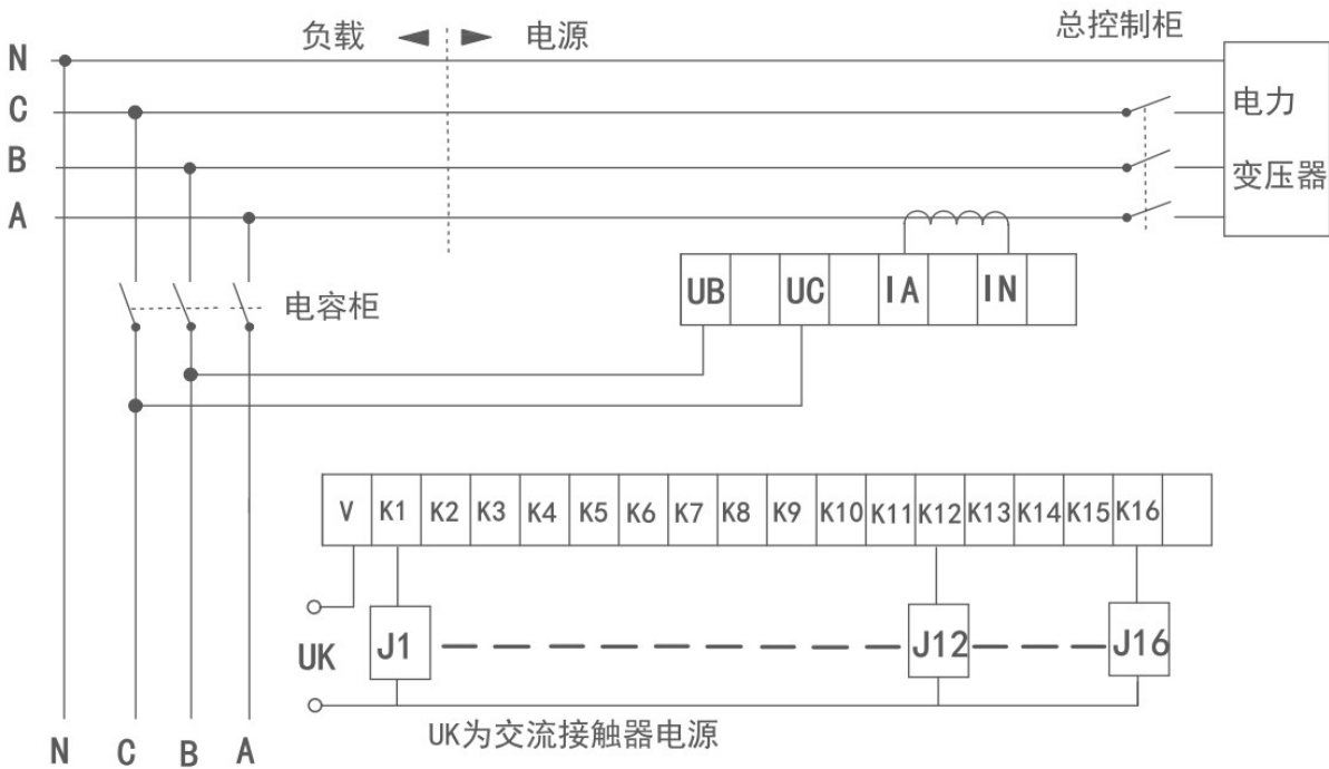
接线图 2 (取样电压 380V)
